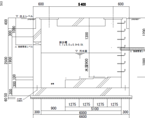
No.2排水ポンプ槽
