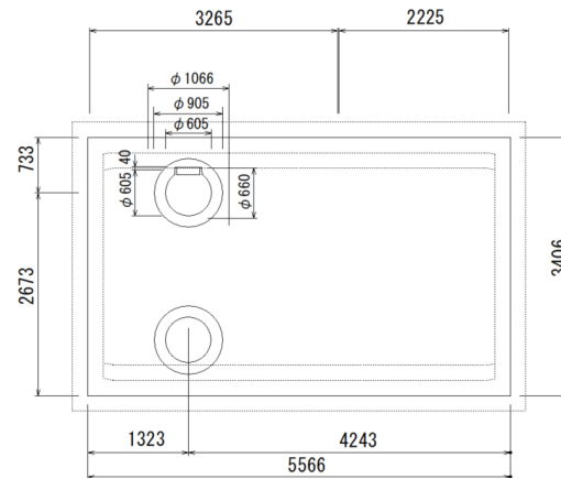
平面図
