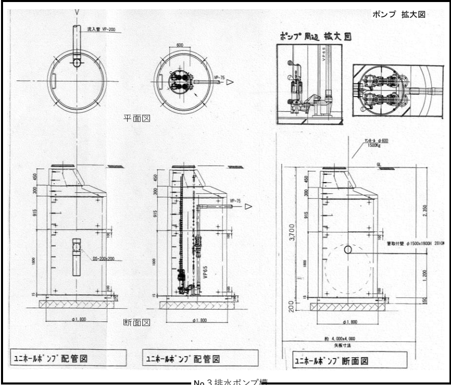
No.3排水ポンプ槽
