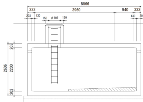
No.4-1排水ポンプ槽
