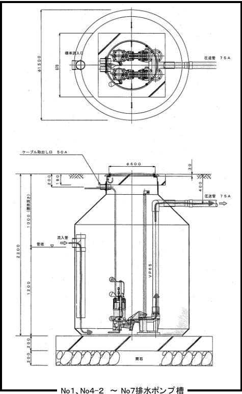
No.1、No.4-2 ~ No.7排水ポンプ槽
