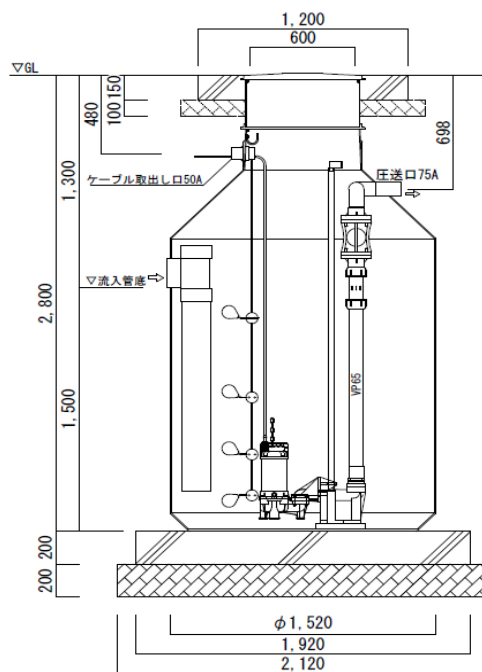
断面図
