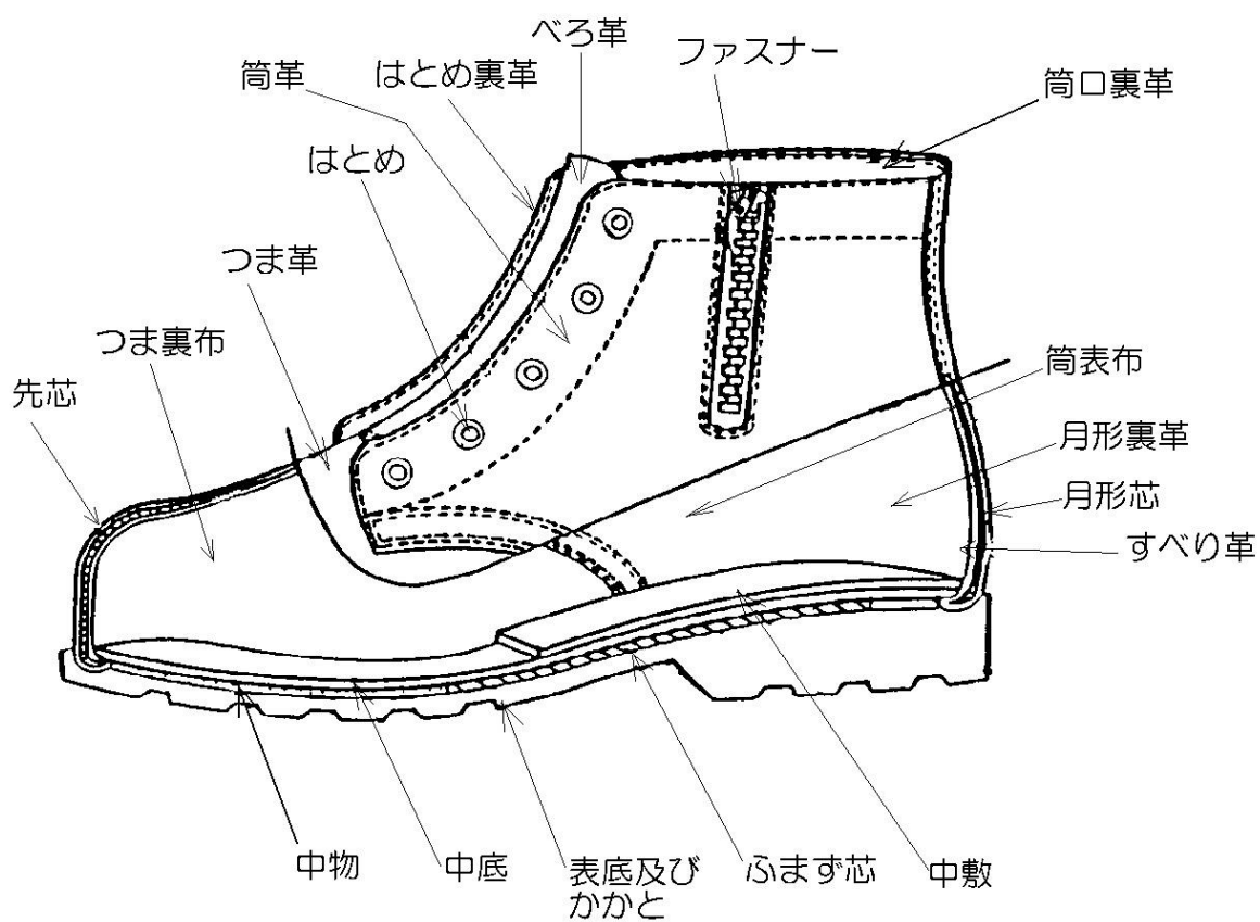
断面図
