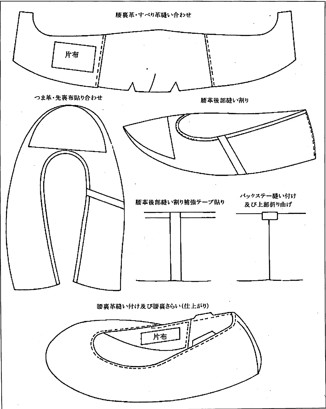
付図9の2（製甲）
