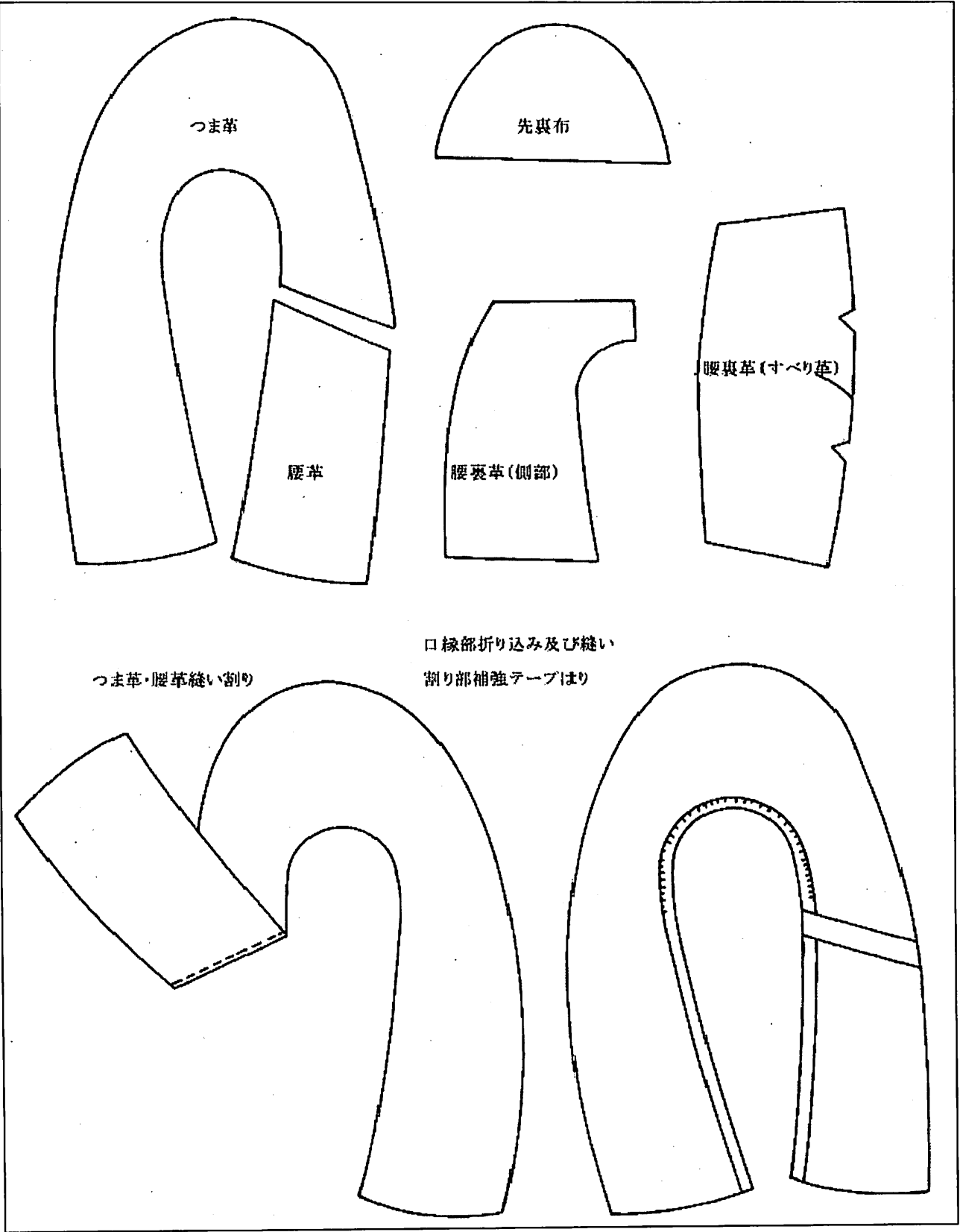
付図9の1 (製甲)
