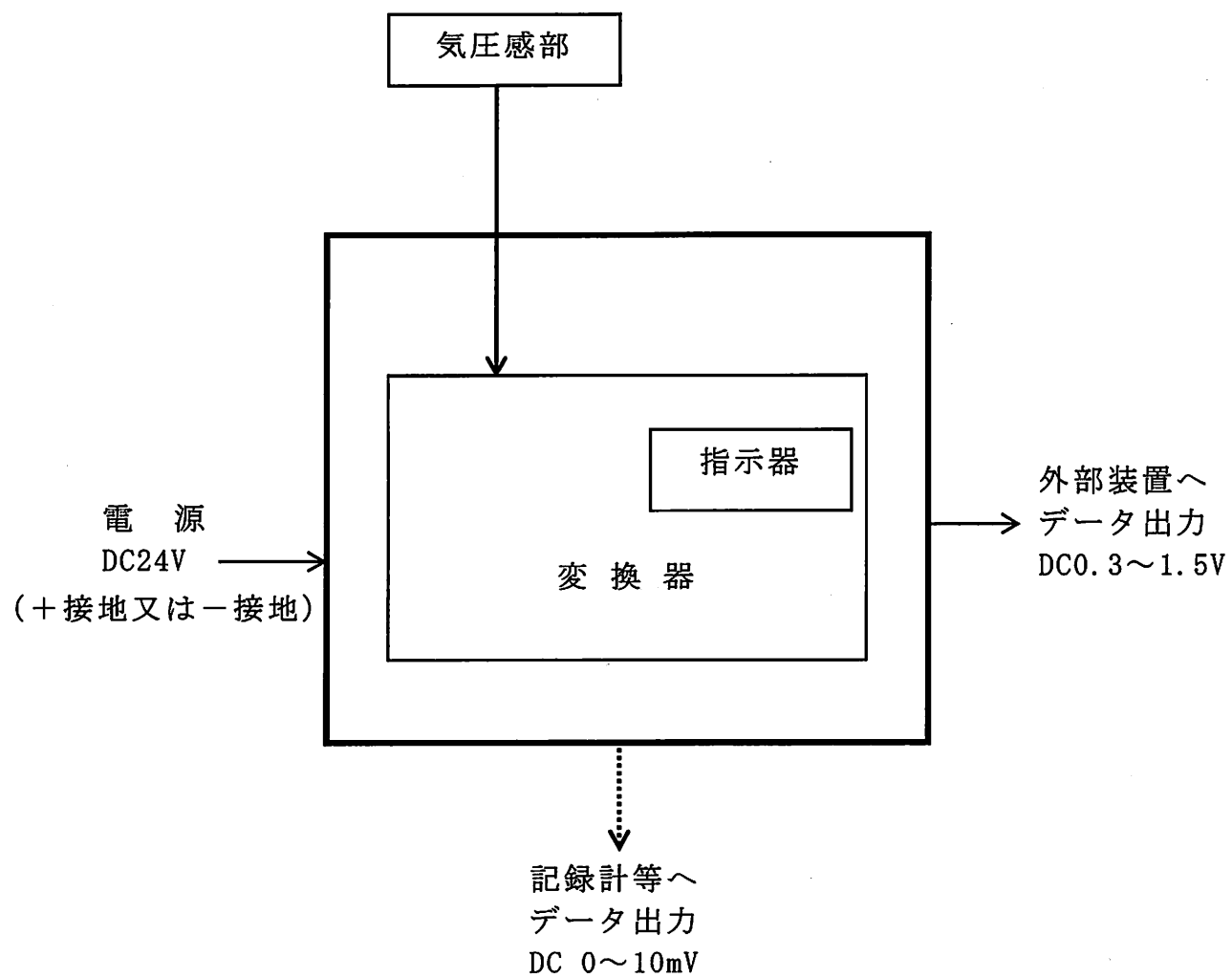
第 1 図 隔測気圧計系統図
