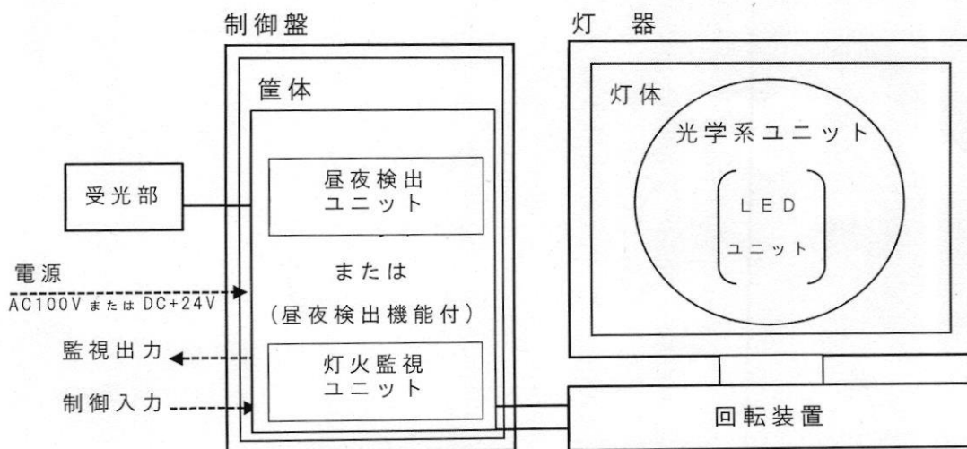
図 1. 系統図
