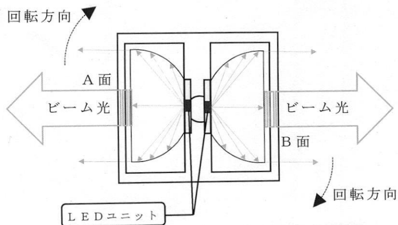
図 2. 灯体内部を上から見た一例
