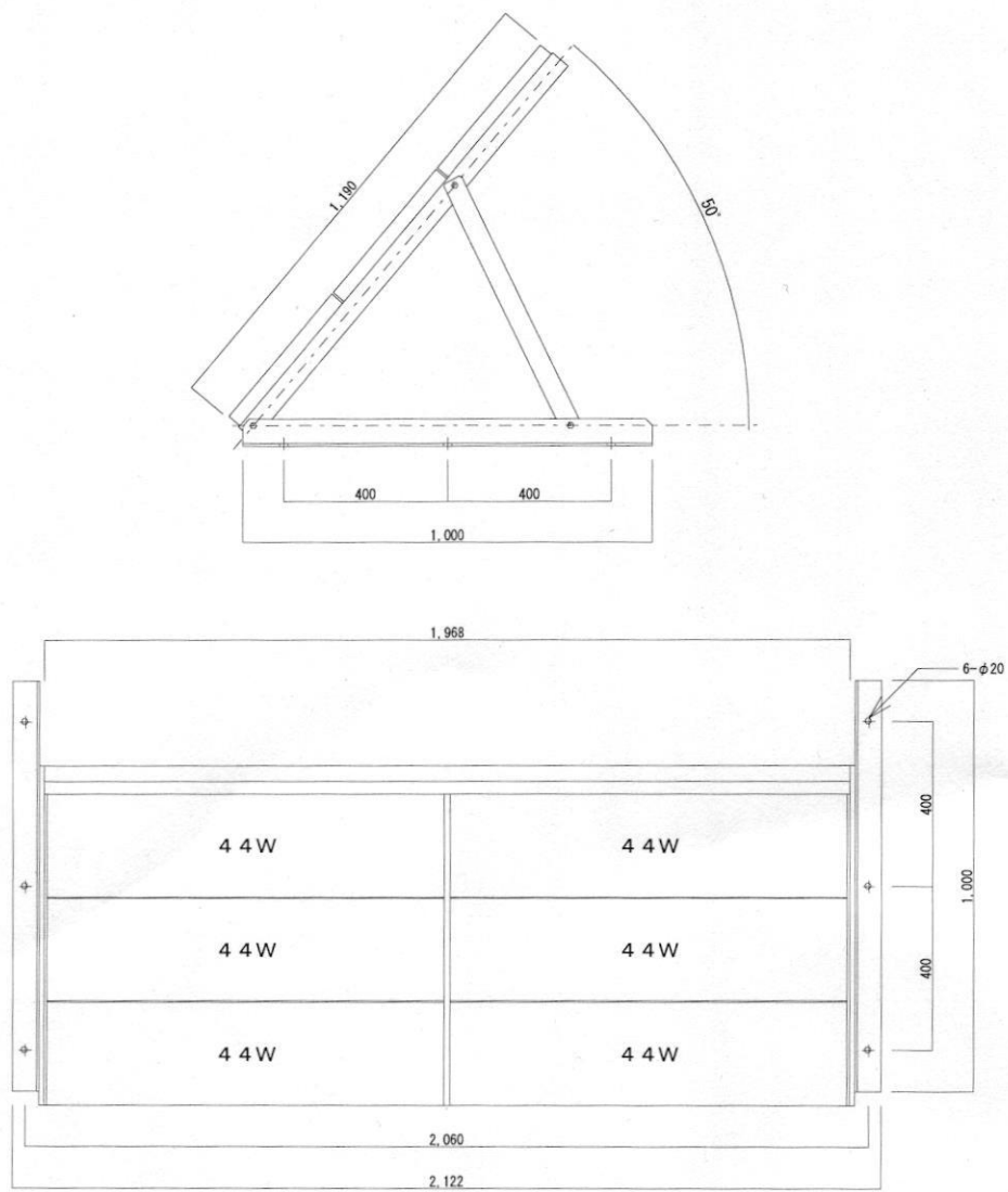
太陽電池架（12Vor24V-264W）
