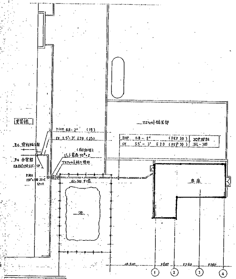
配管図 5/200
