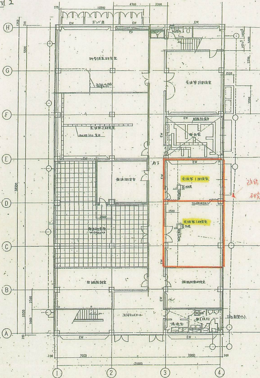
1. 階平面図
