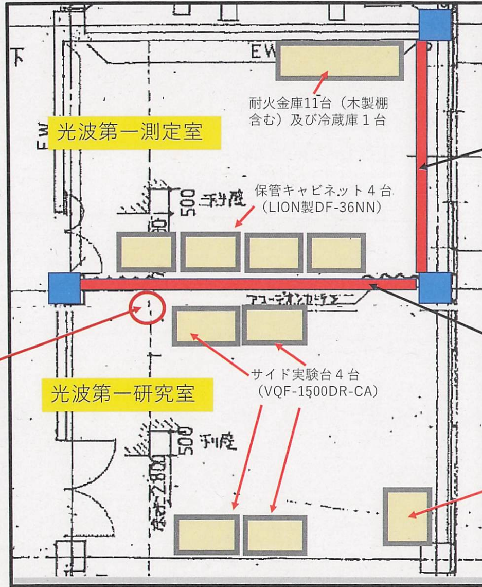
間仕切り壁位置及び什器等設置図
