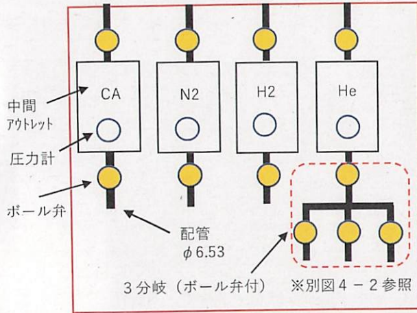
特殊ガス中間アウトレット設置図
