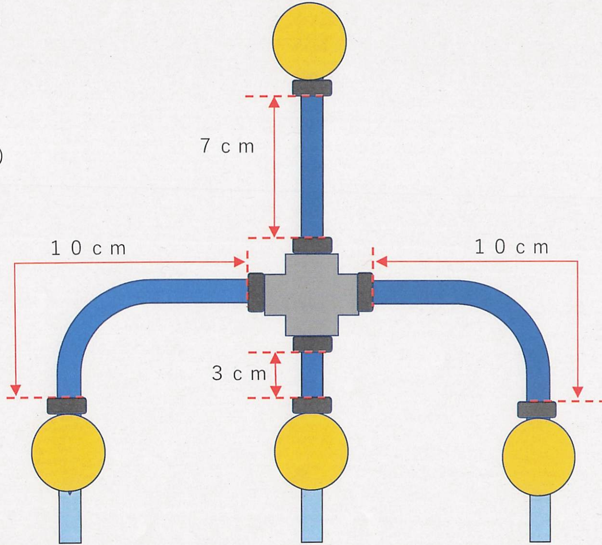
3分岐（ボール弁付）配管図
