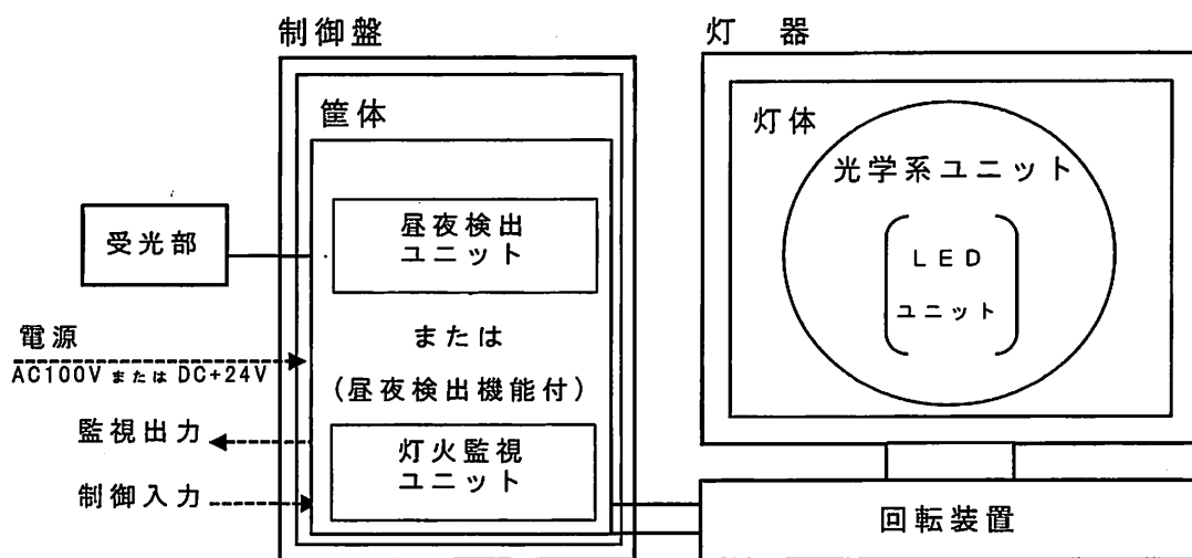
図 1. 系統図
