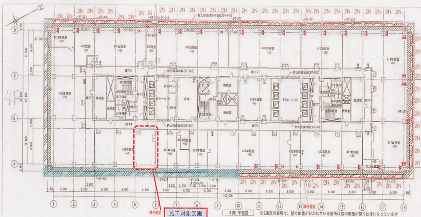
別図1 中央合同庁舎4号館 4階平面図
