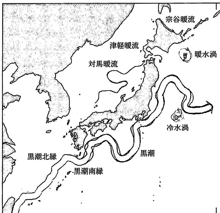
図5. 海流流線の例（黒線：前号の流線、灰線：本号の流線）
