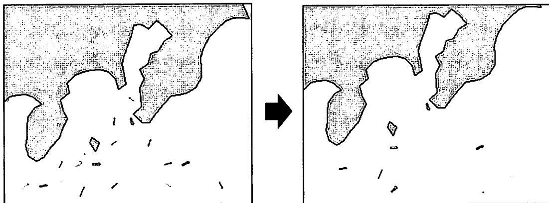
図 6. 平均化した海流矢符の例（左側で不採用にした矢符を右側で非表示にした例）
