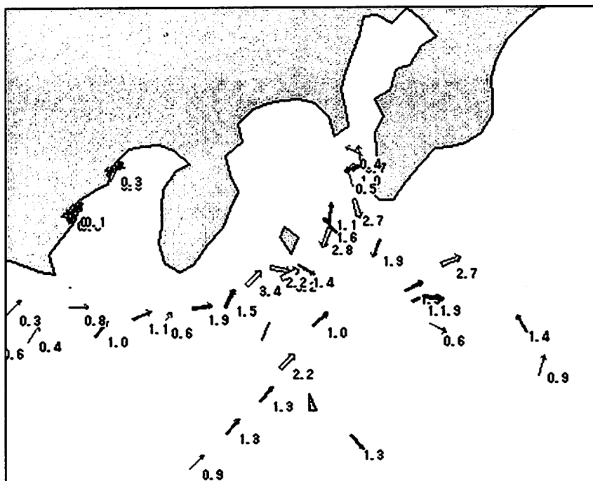
図 3. 海流矢符の表示の例 (矢符の向きは流向で、数字は流速 (単位: ノット) を示す)
