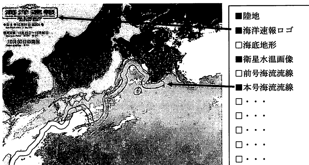
図2. ArcGIS に表示させる画像の例 (■のチェックが入った画像だけ表示される)
