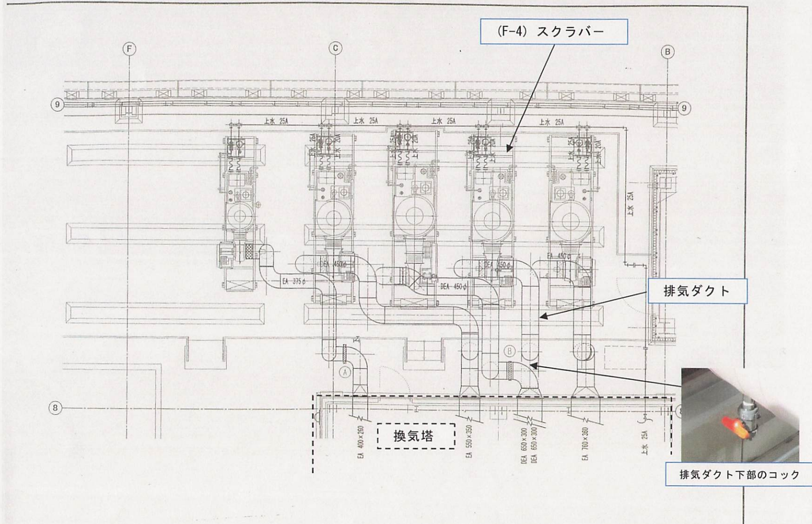
図2 排気ダクト平面図
