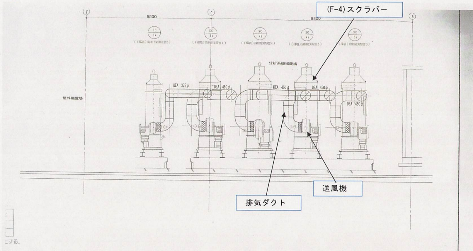
図3 スクラバーと排気ダクト
