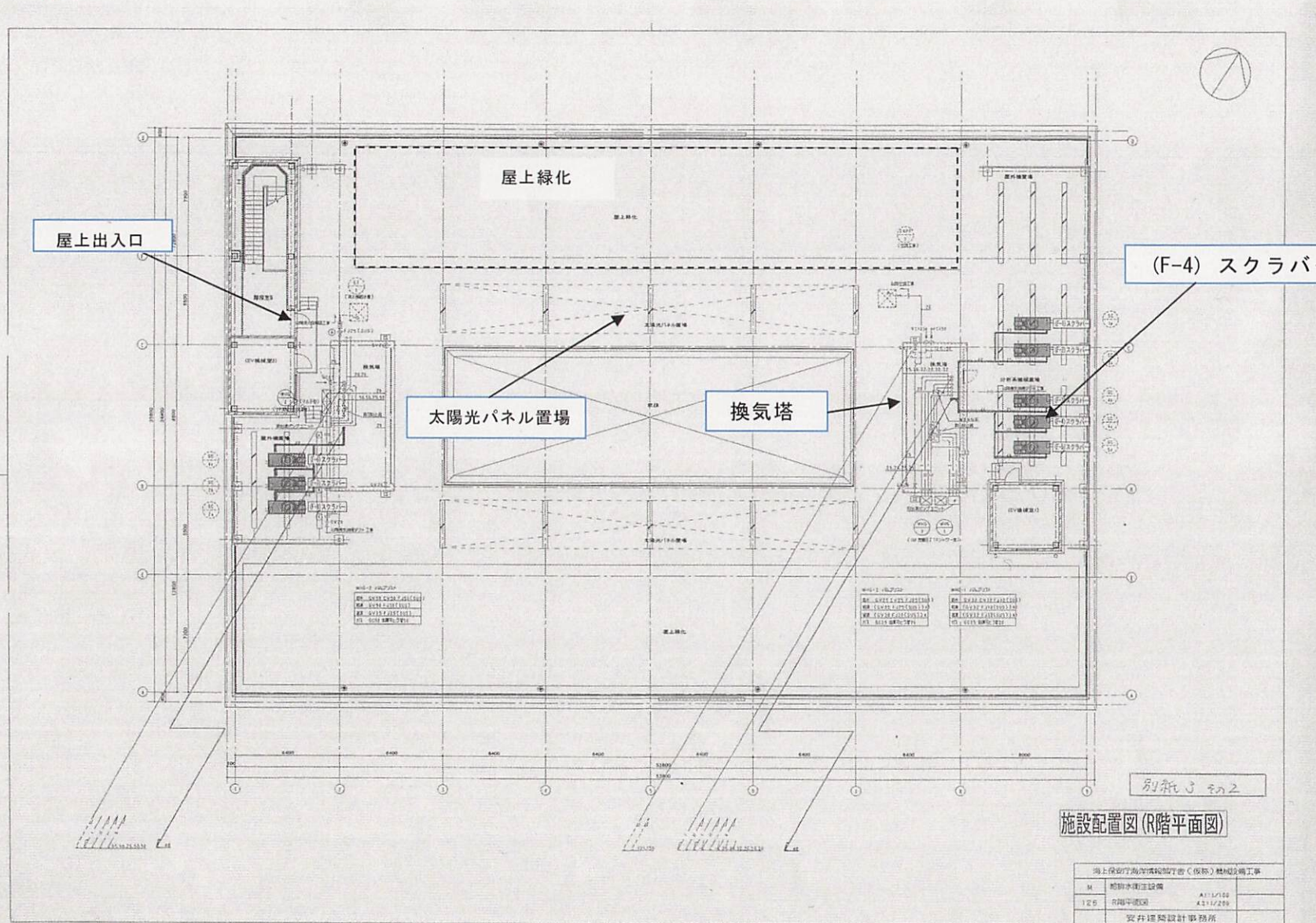
図1 屋上施設配置図
