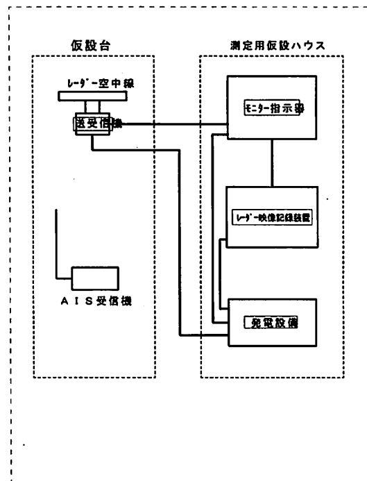
測定用機器系統図
