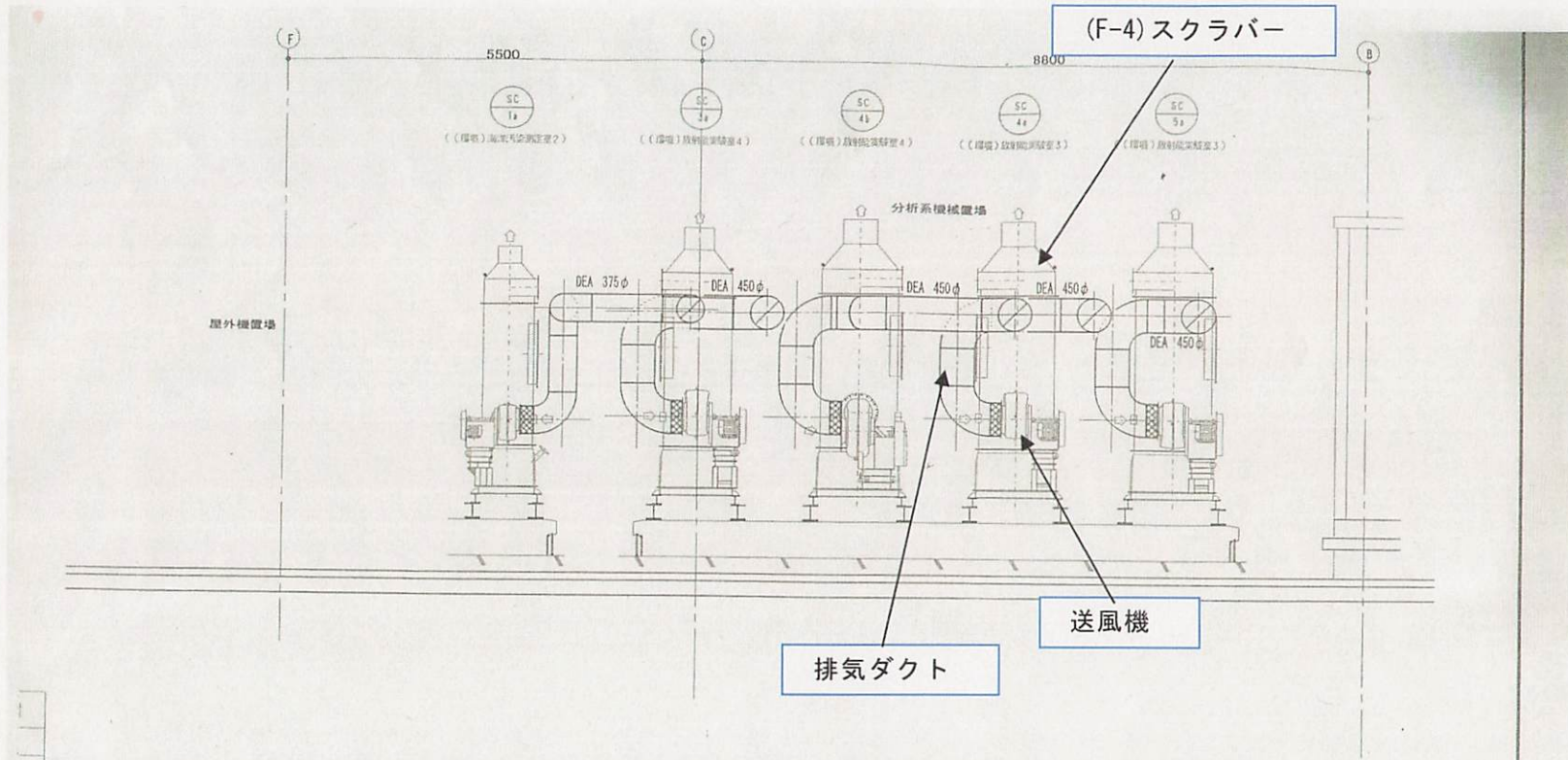
図3 スクラバーと排気ダクト
