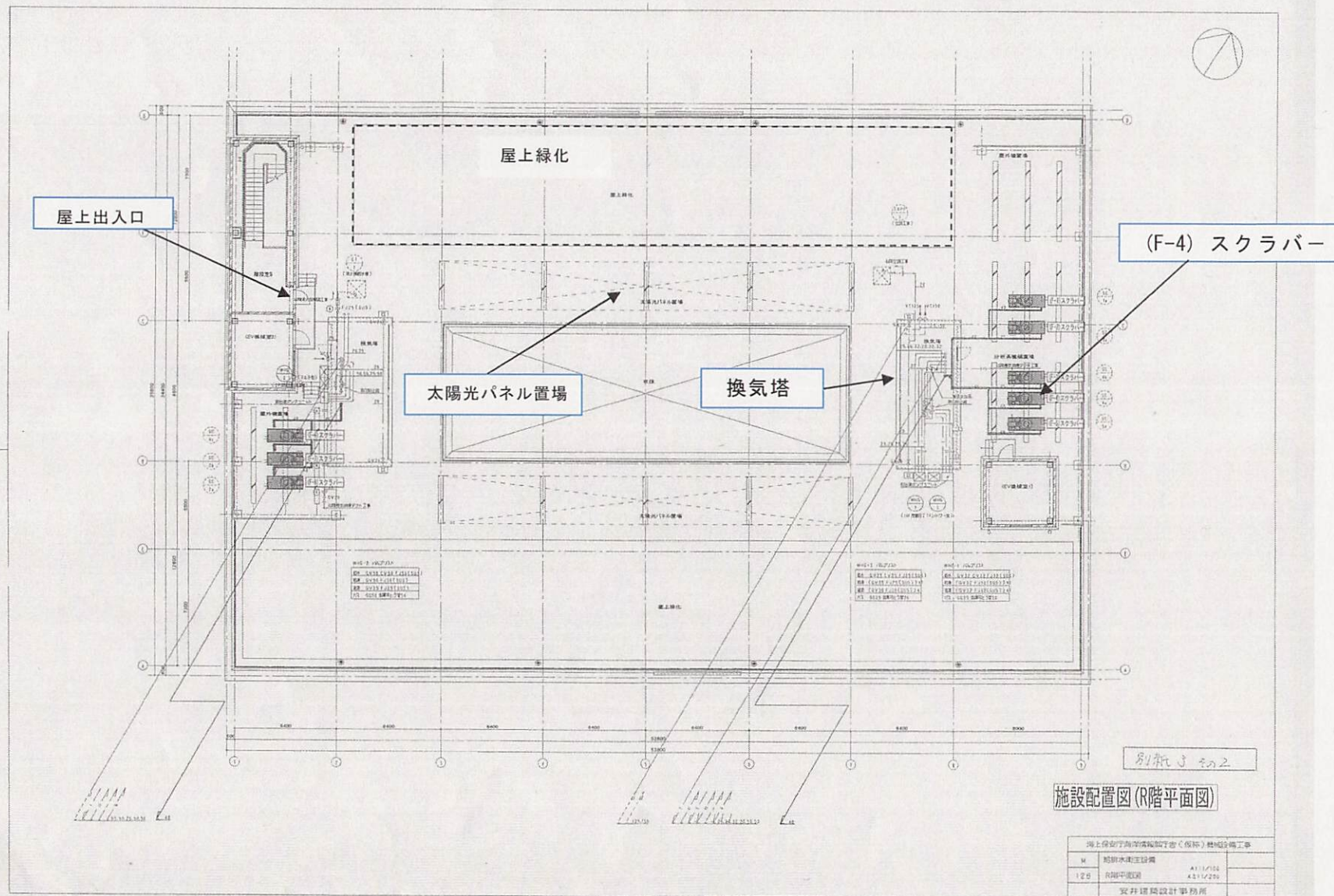
図1 屋上施設配置図
