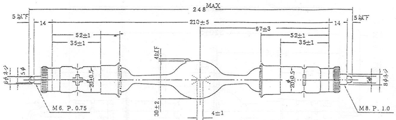
構造寸法図
