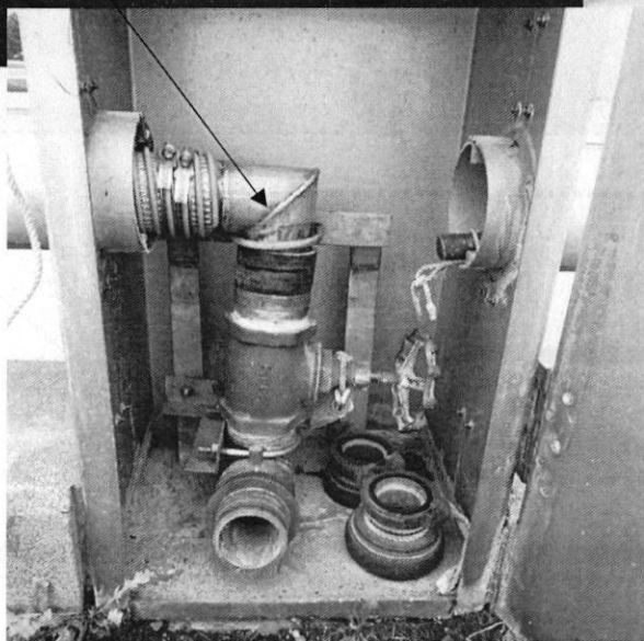
給水栓 ボックス
