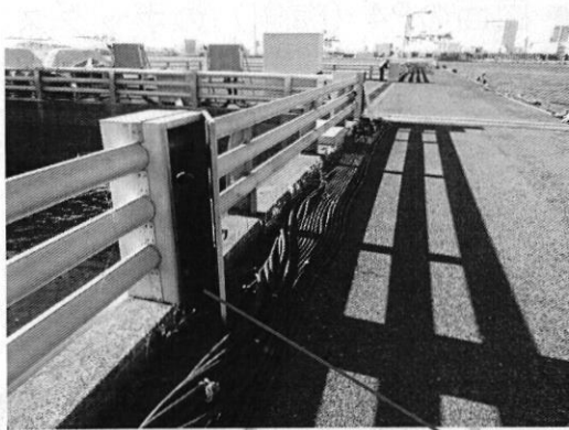
中央の給水栓ボックス
