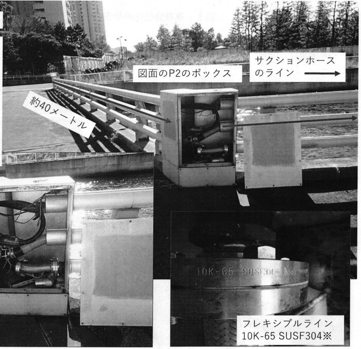
図2 連絡橋海側の状況
