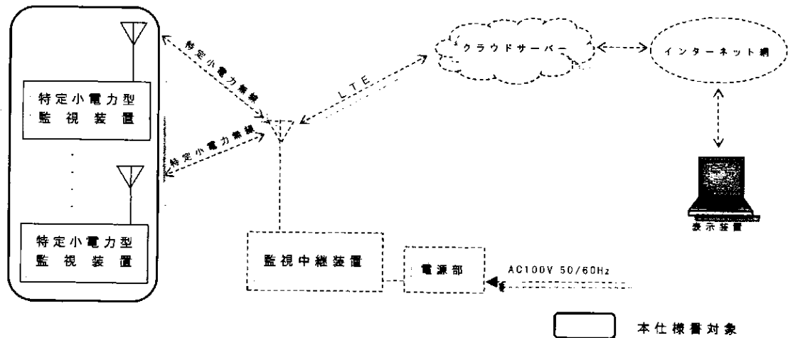
図 1 システム構成図
