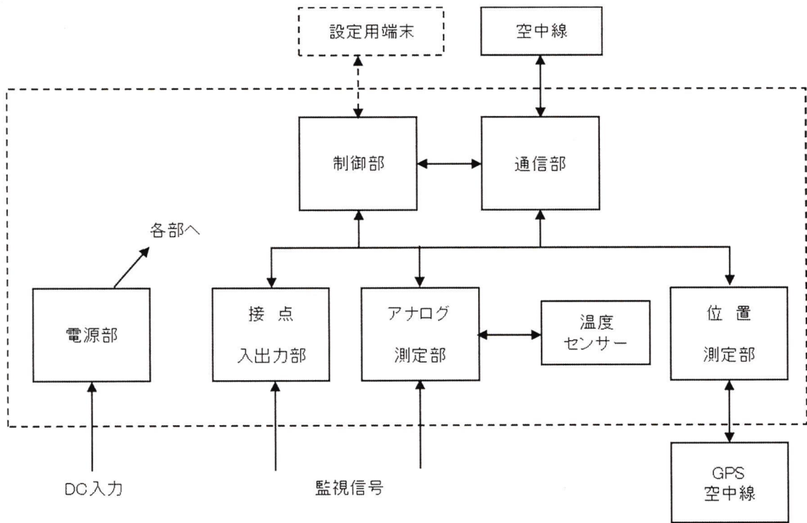
第1図 系統図
