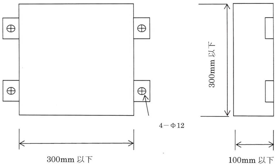
第2図 概観図
