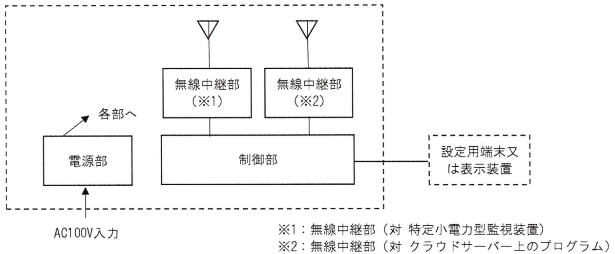
第 1 図 系統図
