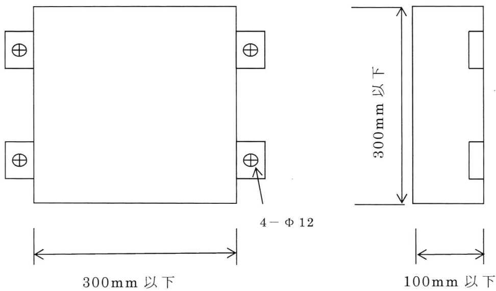
第2図 概観図
