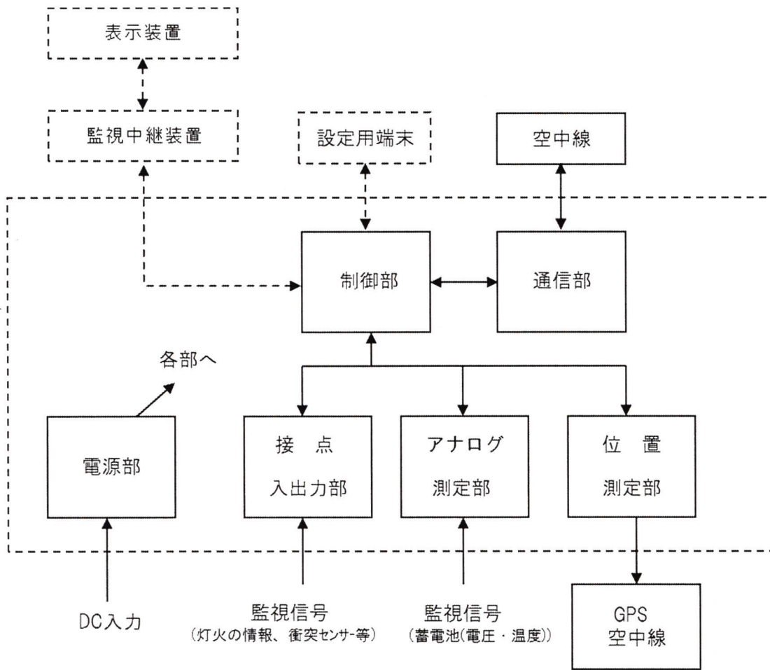
第1図 系統図
