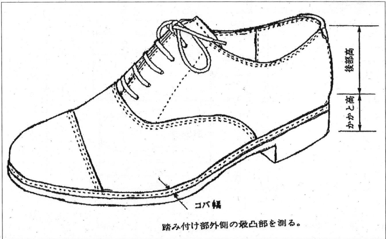
付図1（外観及び各部寸法）
