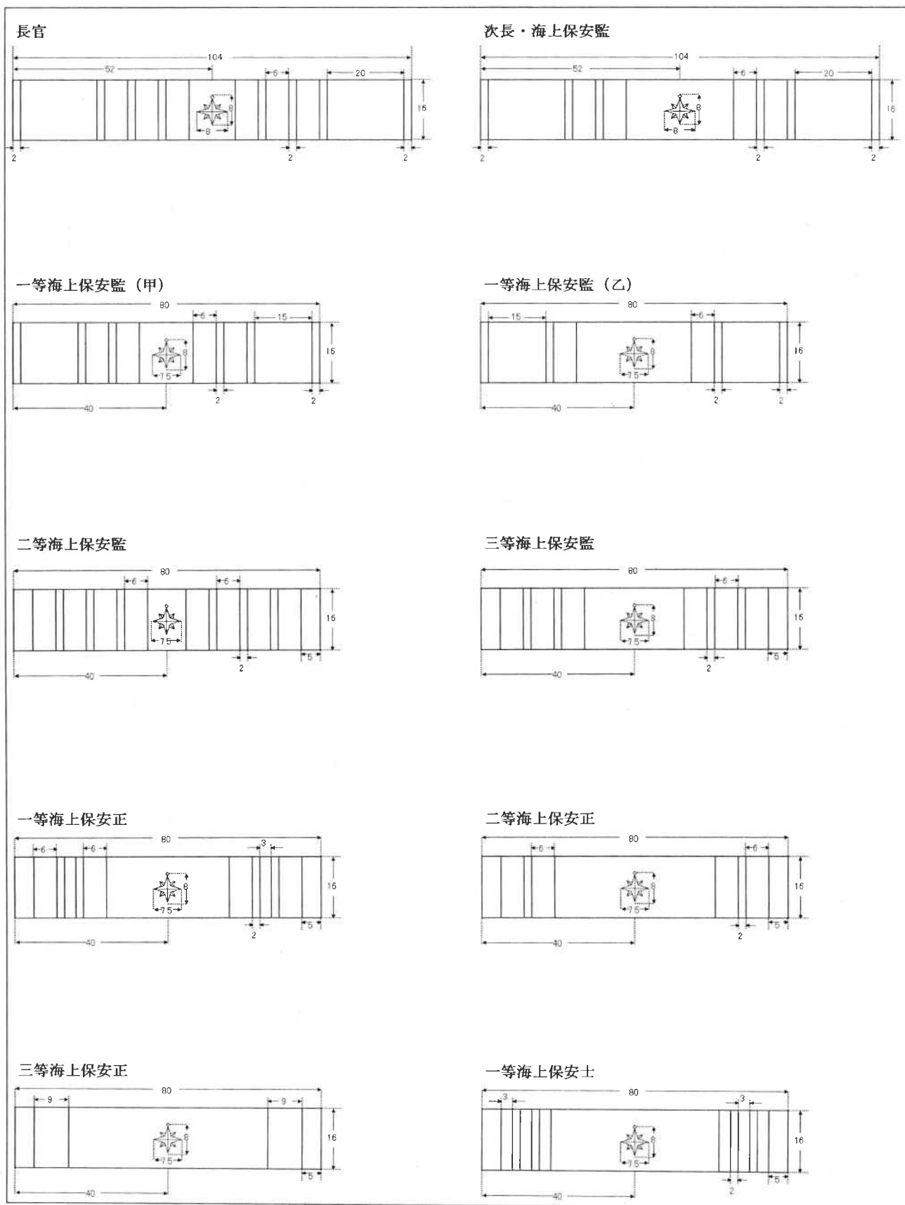
別図 2 (数字は寸法を示し単位はミリメートル (mm) とする。)
