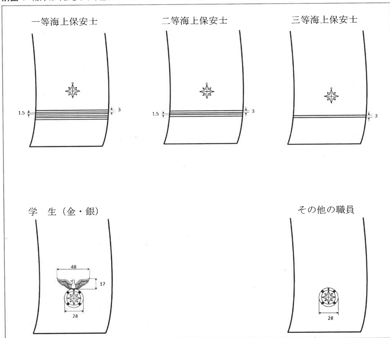
別図 4 (数字は寸法を示し単位はミリメートル (mm) とする。)
