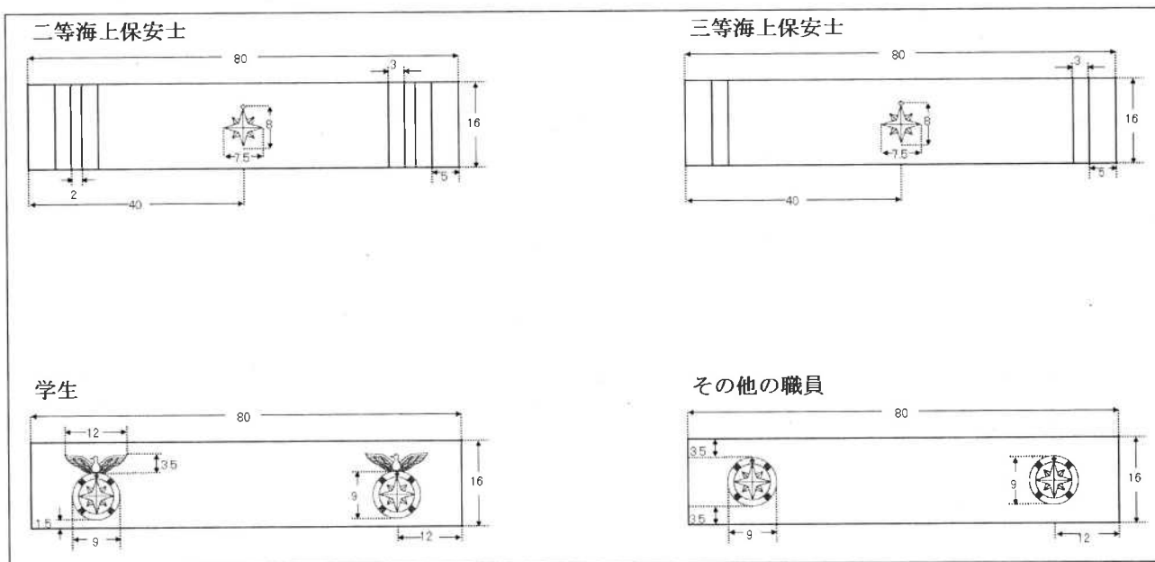
別図 3 (数字は寸法を示し単位はミリメートル (mm) とする。)
