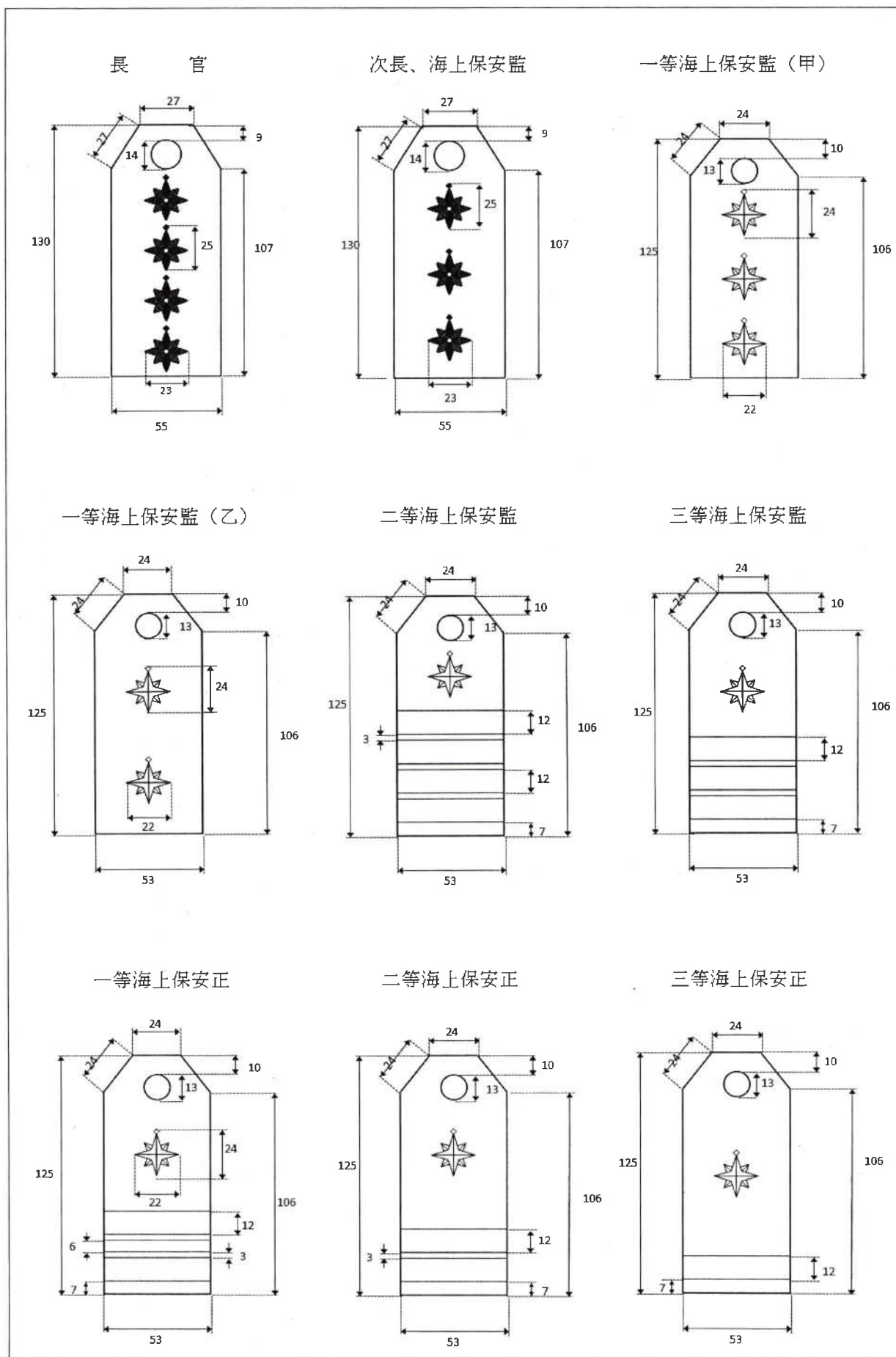
別図 3 (数字は寸法を示し単位はミリメートル (mm) とする。)
