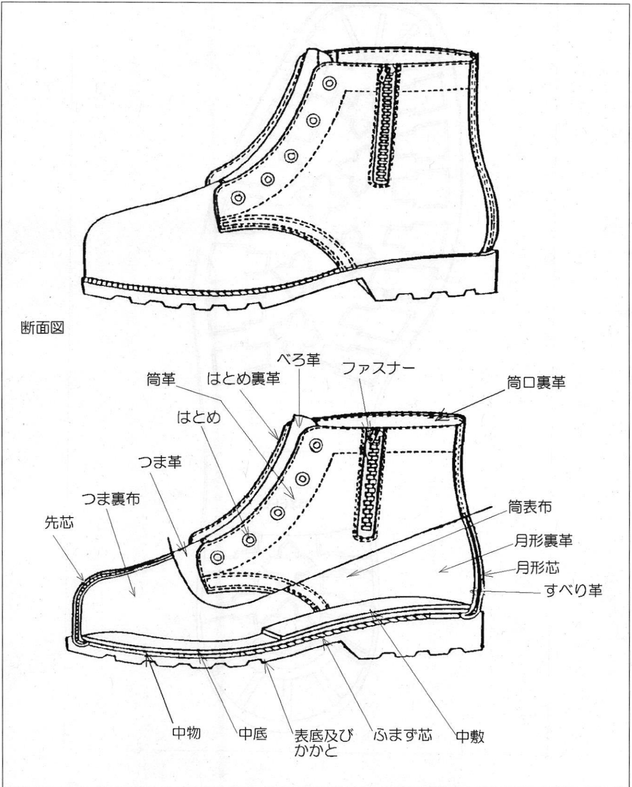
図2 (航空ぐつ) 参考意匠図
