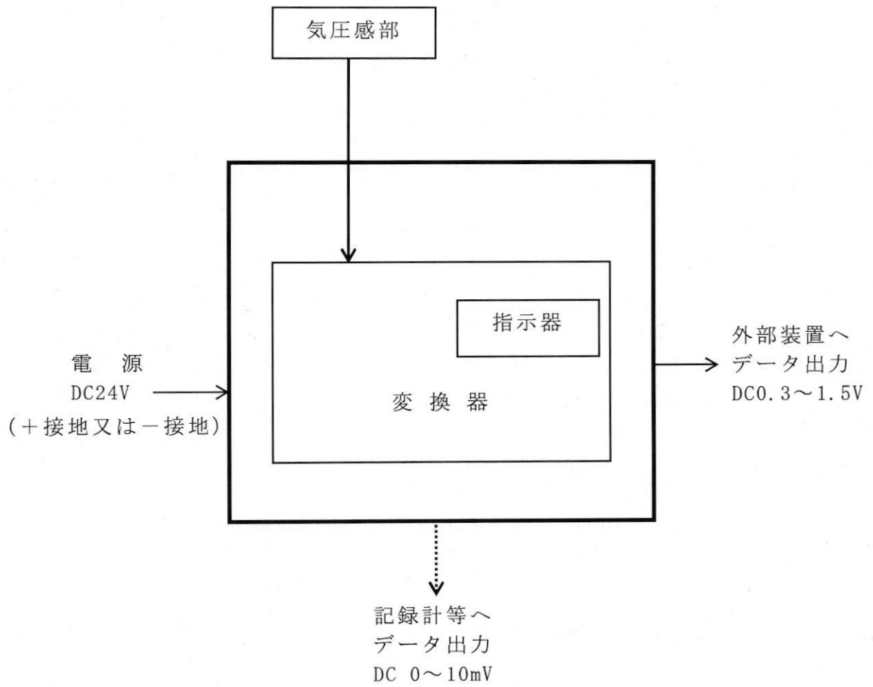
第1図 隔測気圧計系統図
