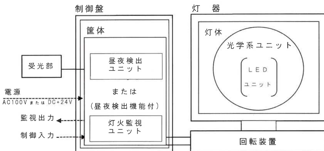
図 1. 系統図
