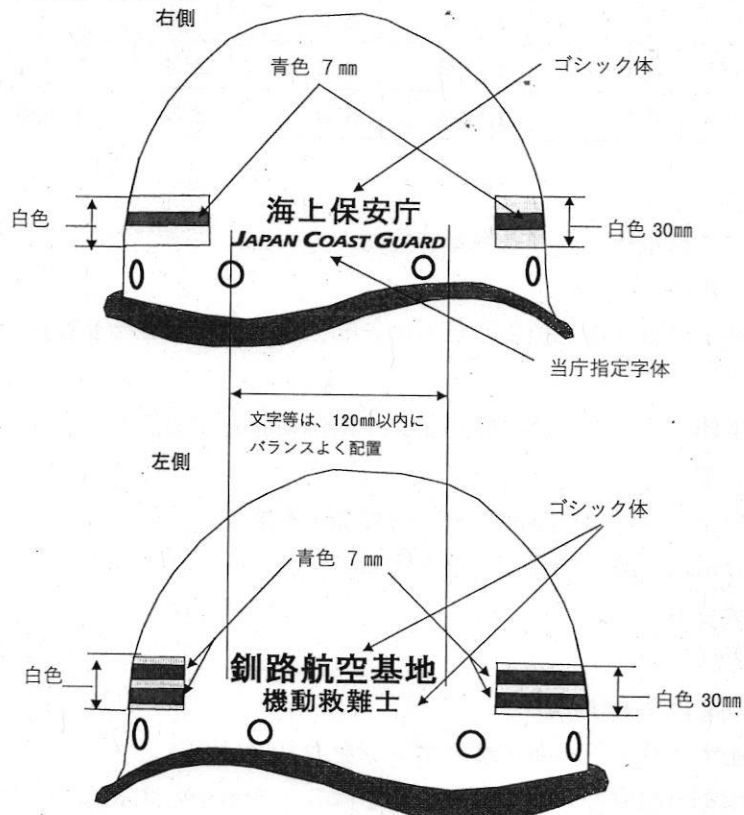
保安帽表示（階級線1本及び2本）
