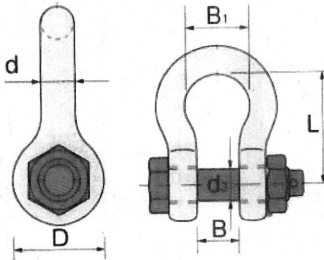
寸法図
