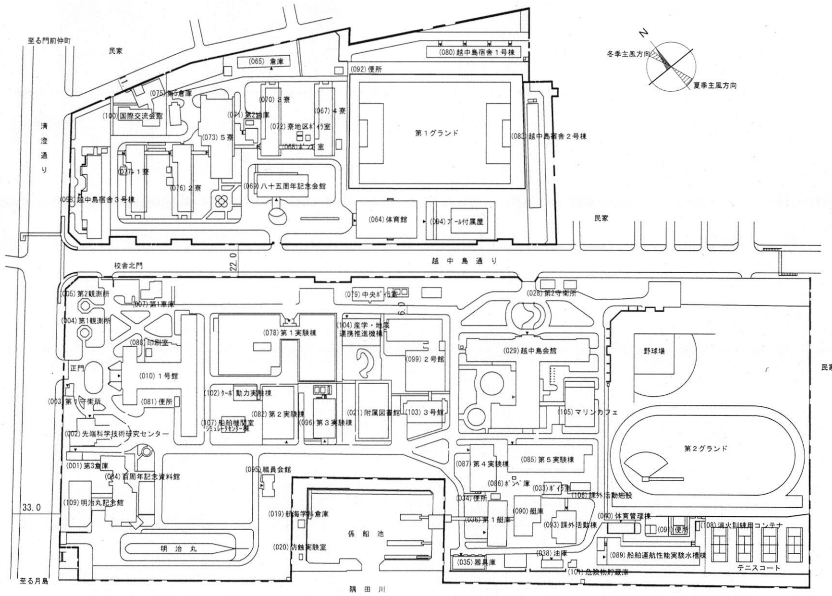
越中島キャンパス配置図 縮尺 S=1/2500
