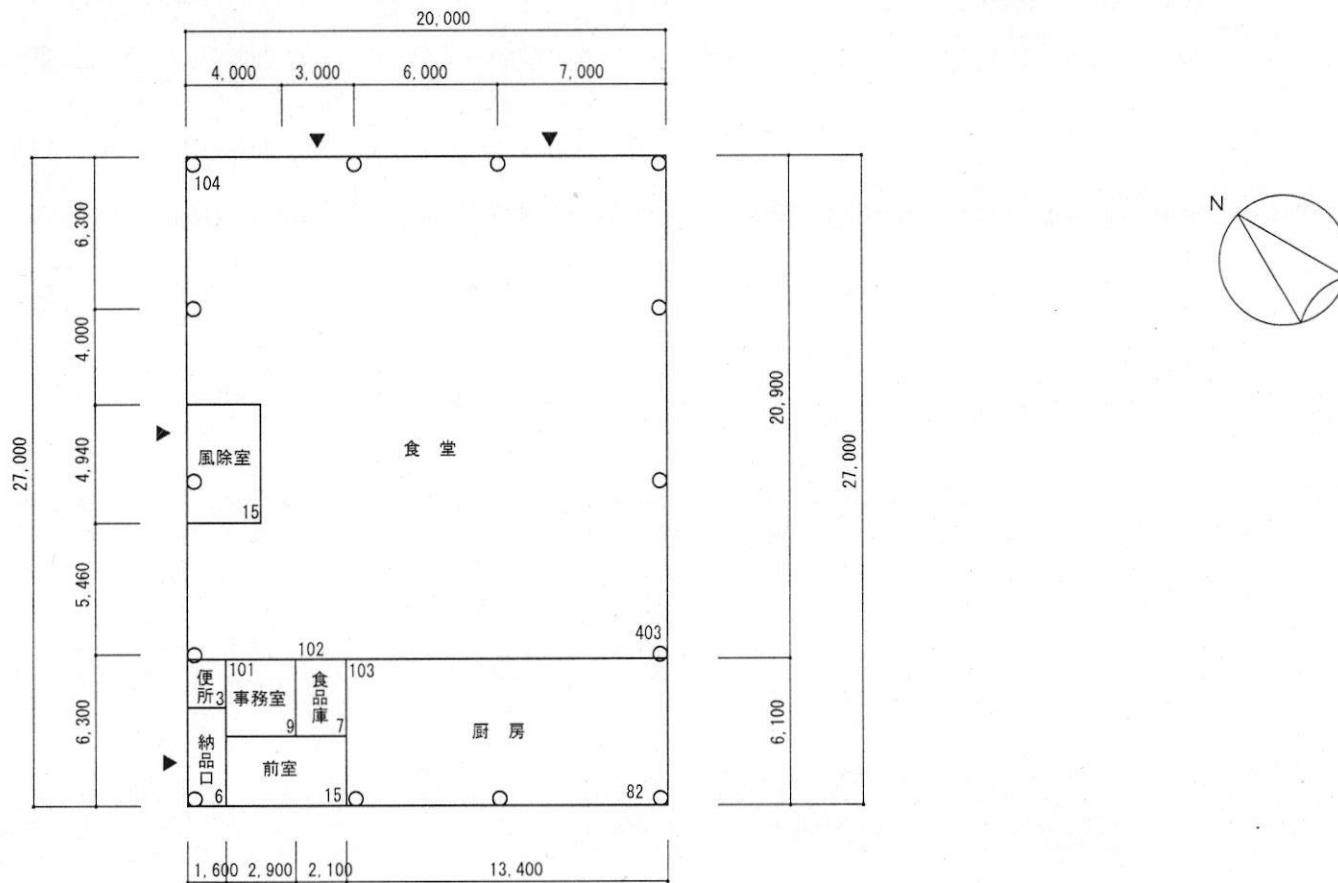
マリン・カフェ 1階平面図 S=1/300 540m 2
