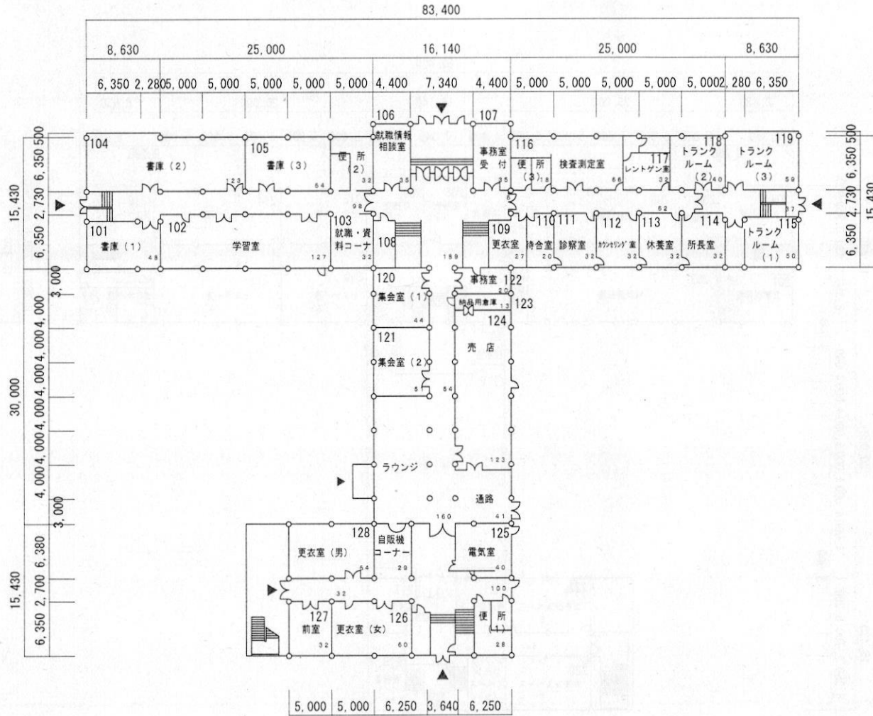
越中島会館 1階平面図 S=1/600 2,233㎡
