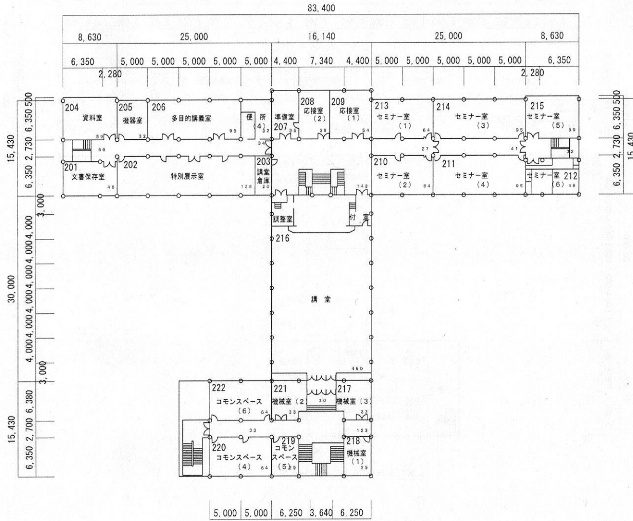
越中島会館 2階平面図 S=1/600 2,223㎡
