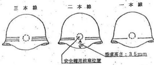
別図3 安全帽前章及び周章の位置
