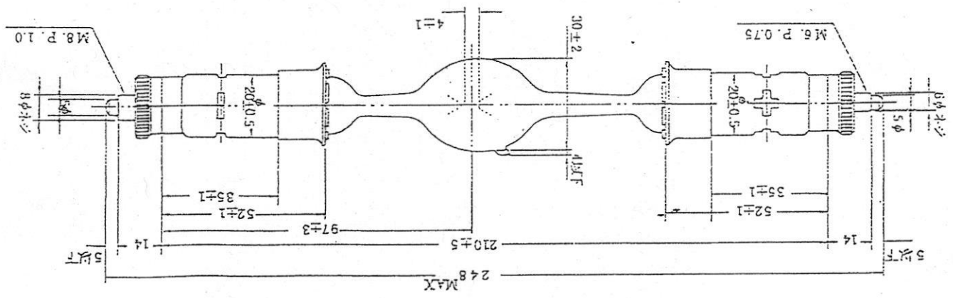
構造寸法図
