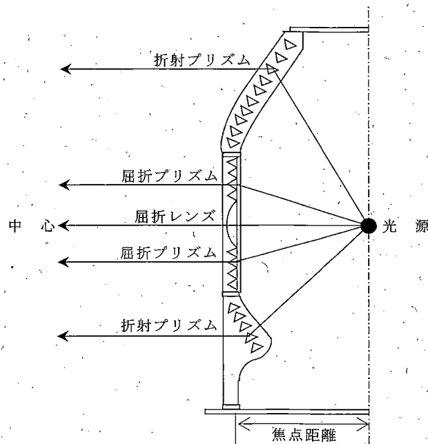
図. フレネルレンズの断面
