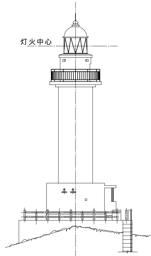
立面図
