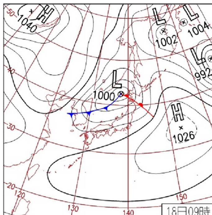
春一番の時の天気図 例
