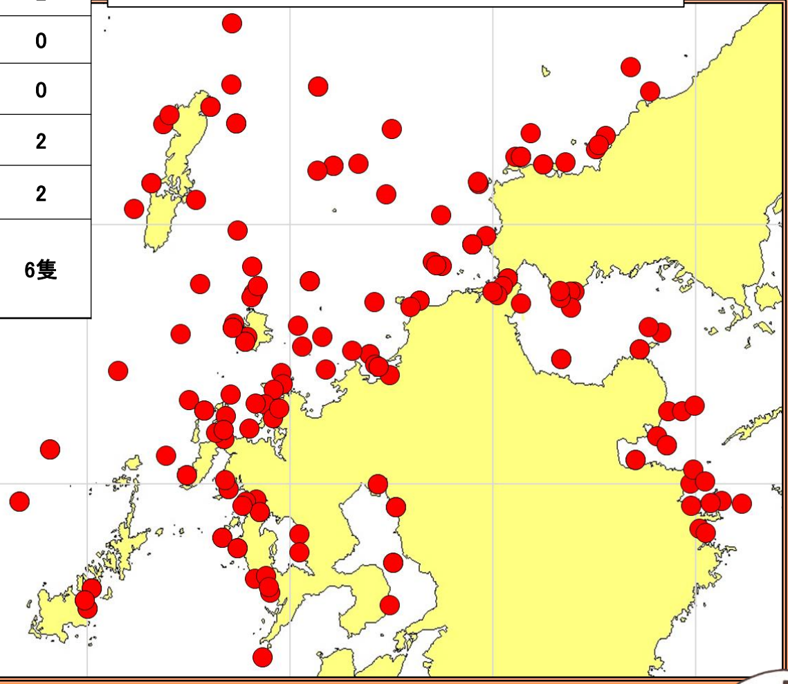
漁船の衝突海難発生位置 (平成28年から令和2年)
