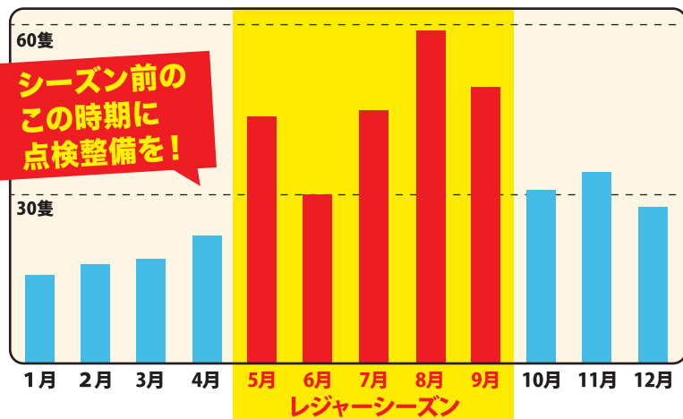
プレジャーボートによる機関故障海難の月別発生状況(過去10年)
