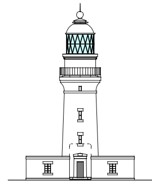
灯台姿図 1 / 500
