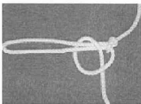
④ もう一方の端末側のロープにもヒッチをかける
