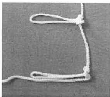
⑦ 最後の段はヒッチを1回のみとし、アイに沿わせる
