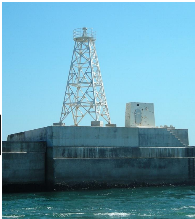
鹿島港南防波堤灯台の全景
